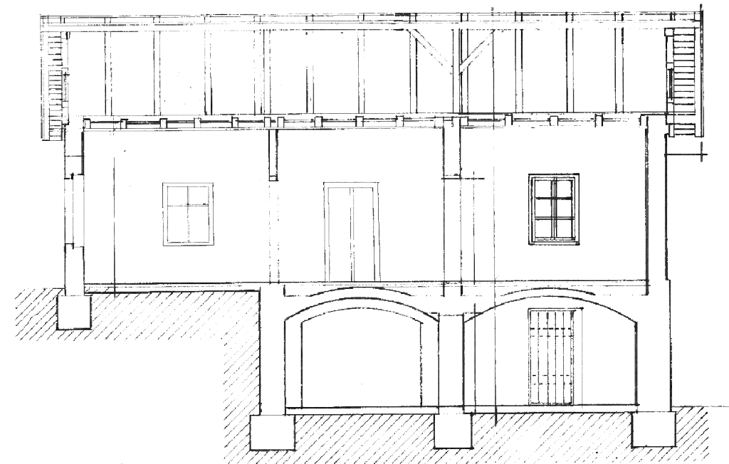
ŘEZ A.B.
