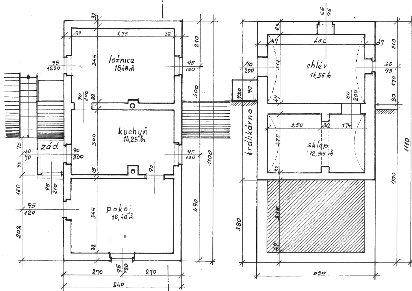
Půdorys
