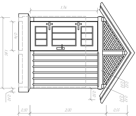
Stirn-Ansicht
